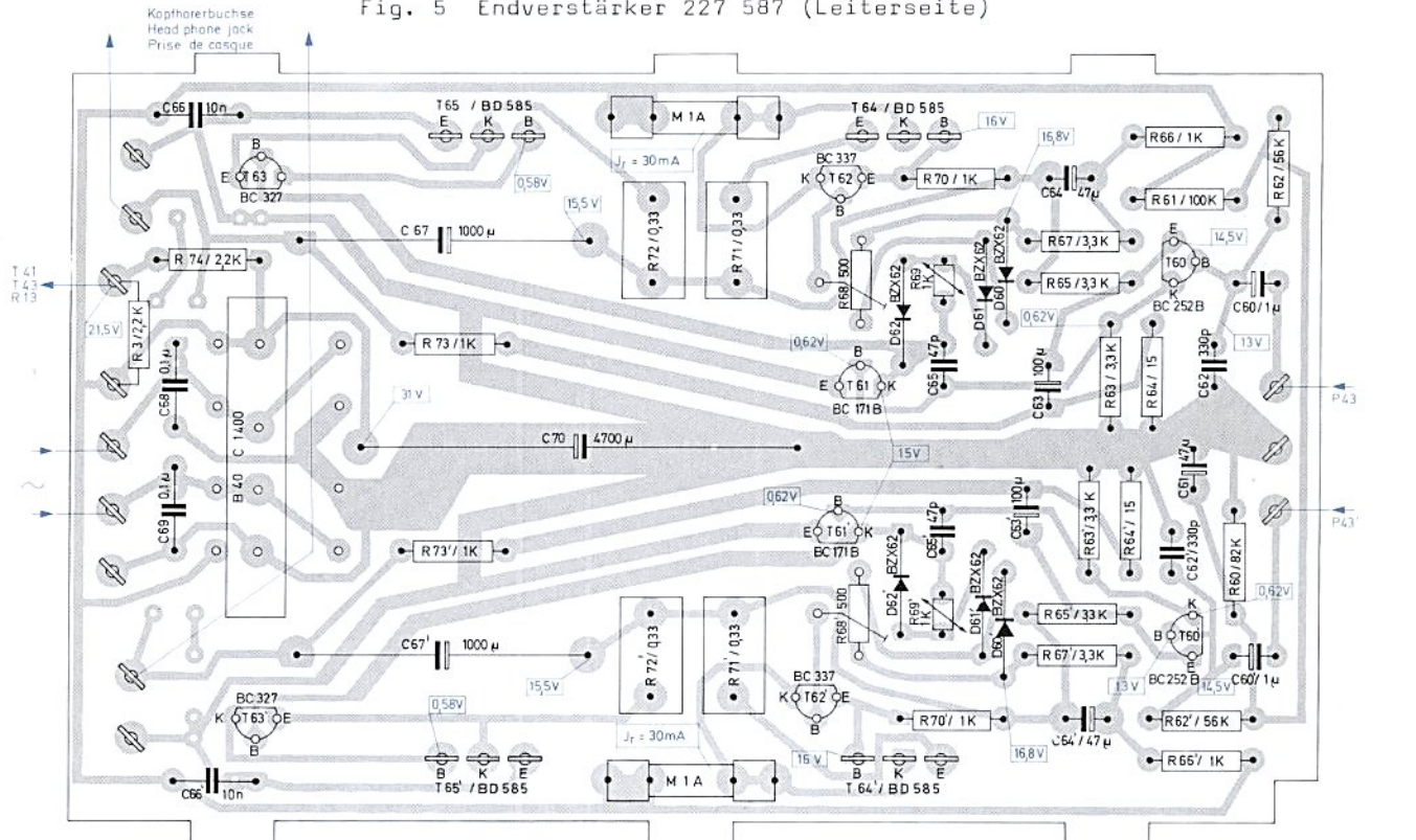
Fig. 5 Endverstärker 227 587 (Leiterseite)
